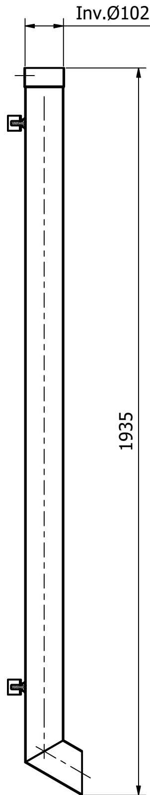
A-A ( 1:10 )
