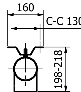
B ( 1:10 )
